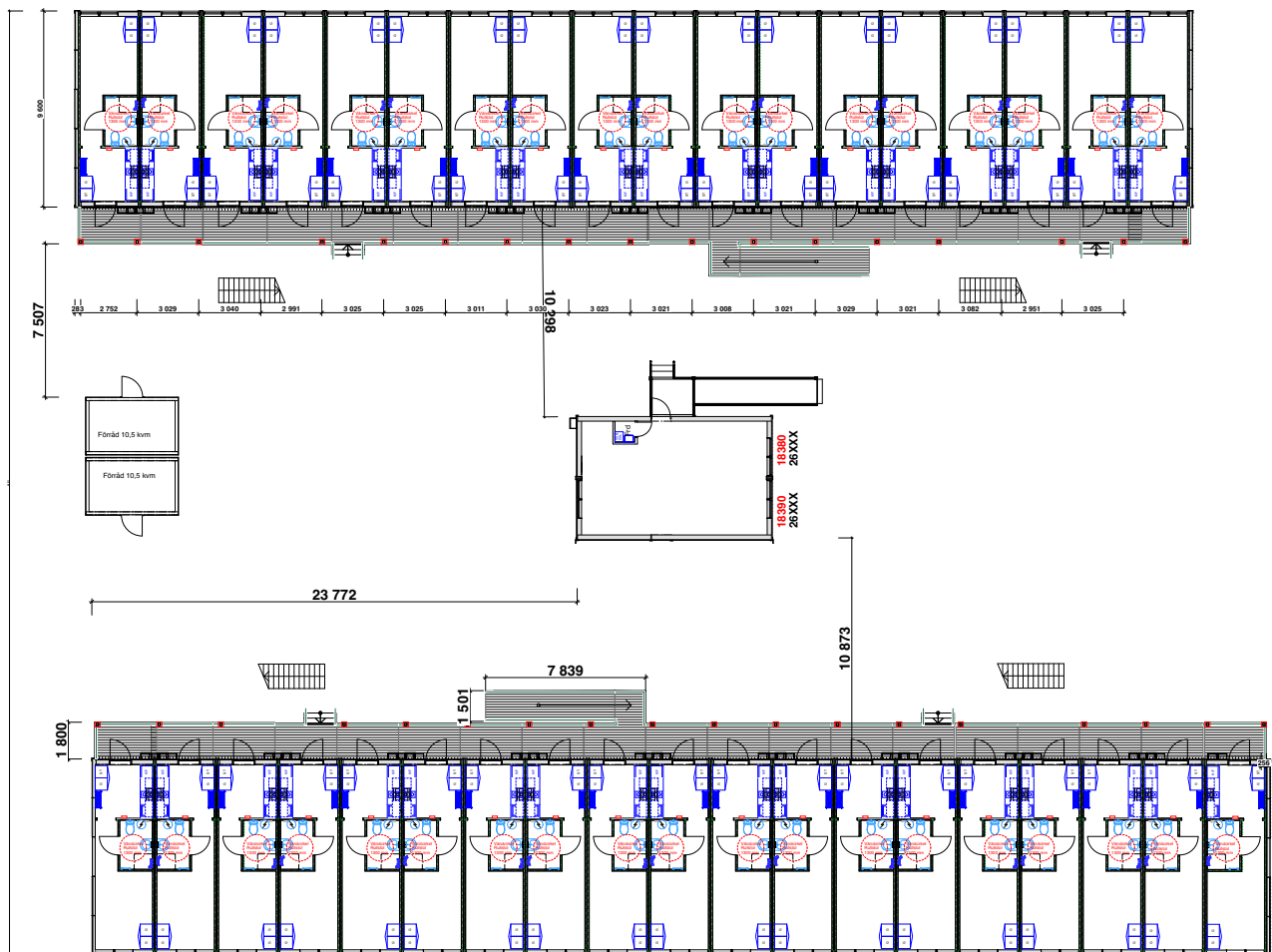
PLANRITNING
